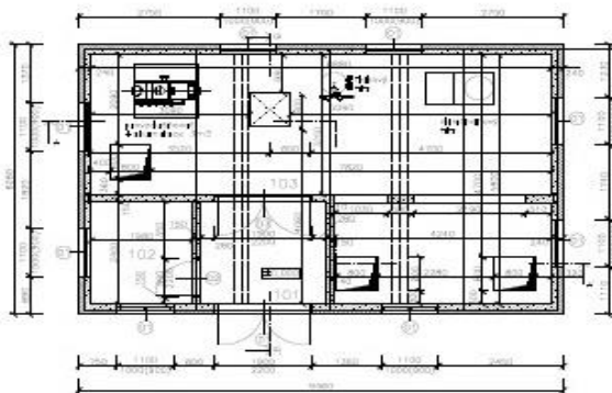
BÚDORYS 1.NP
