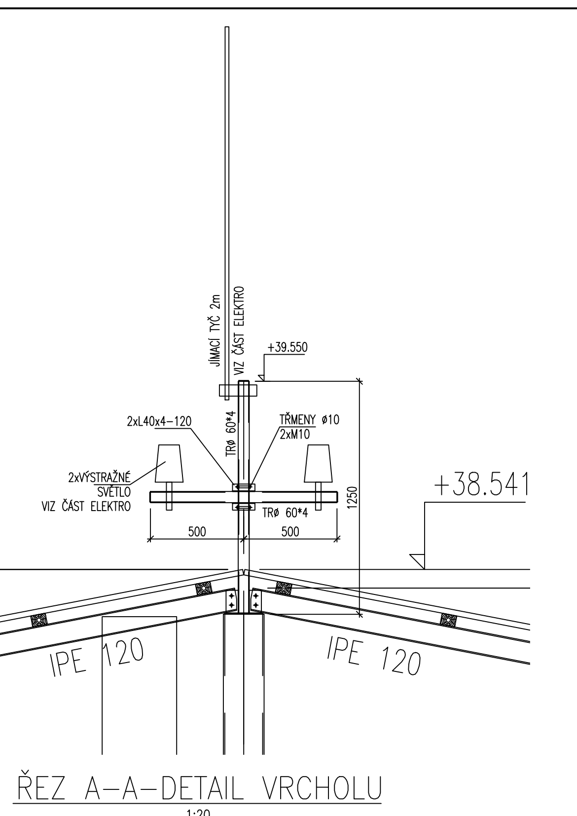
ŘEZ A-A-DETAIL VRCHOLU
