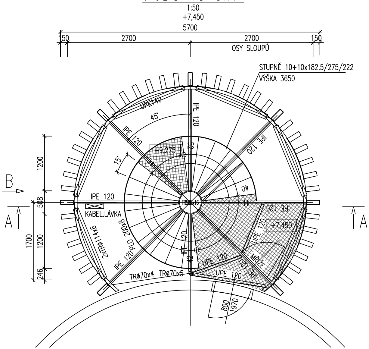
PŮDORYS 2.NP
