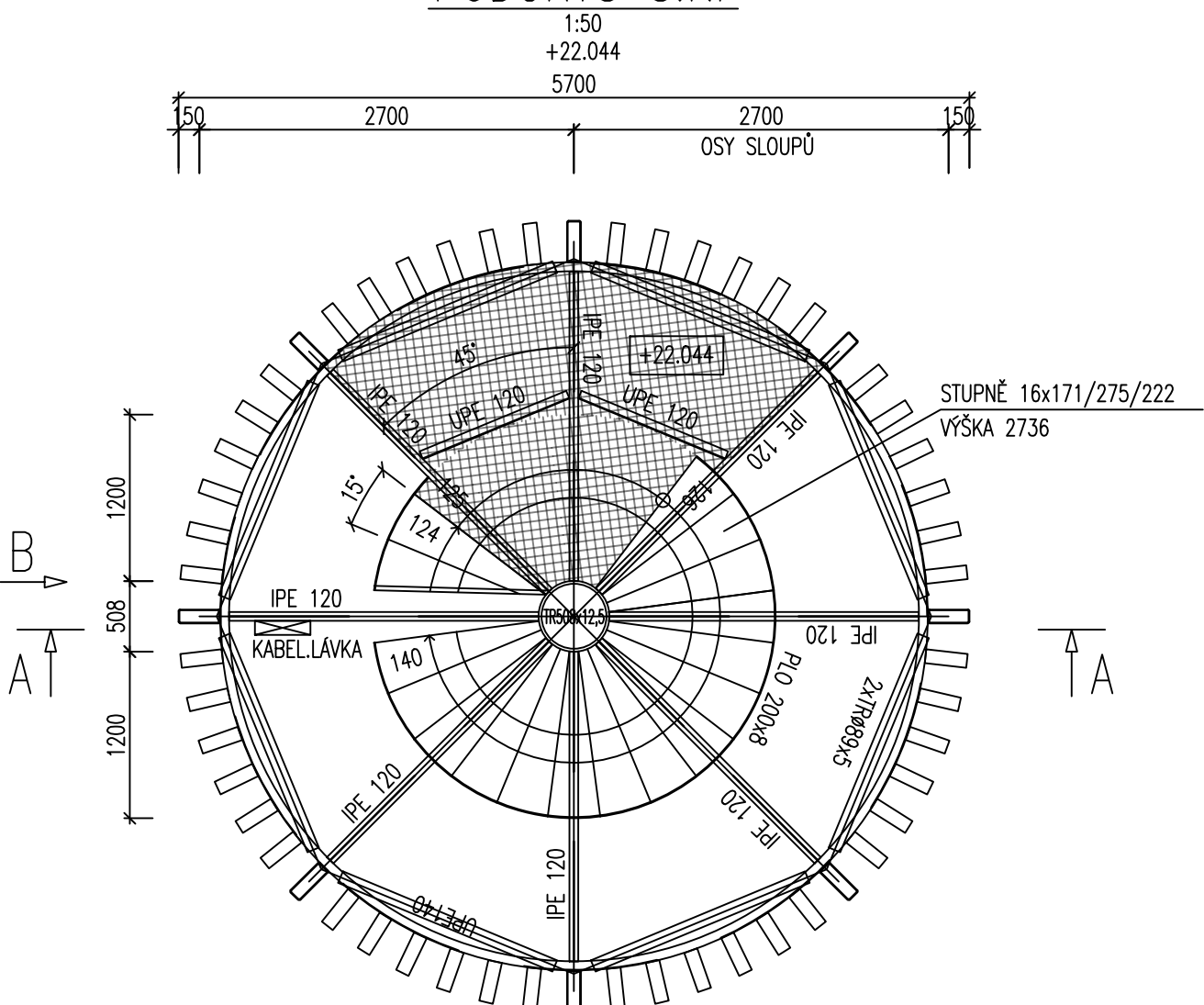
PŮDORYS 8.NP
