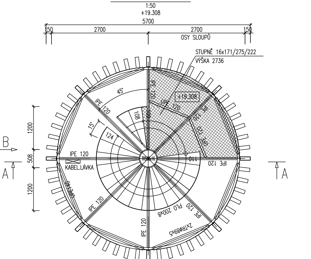
PŮDORYS 7.NP
