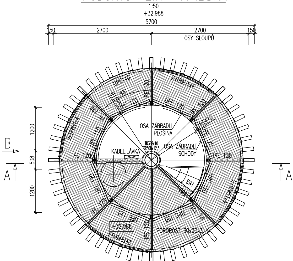
PŮDORYS 12.NP-VYHLÍDKA
