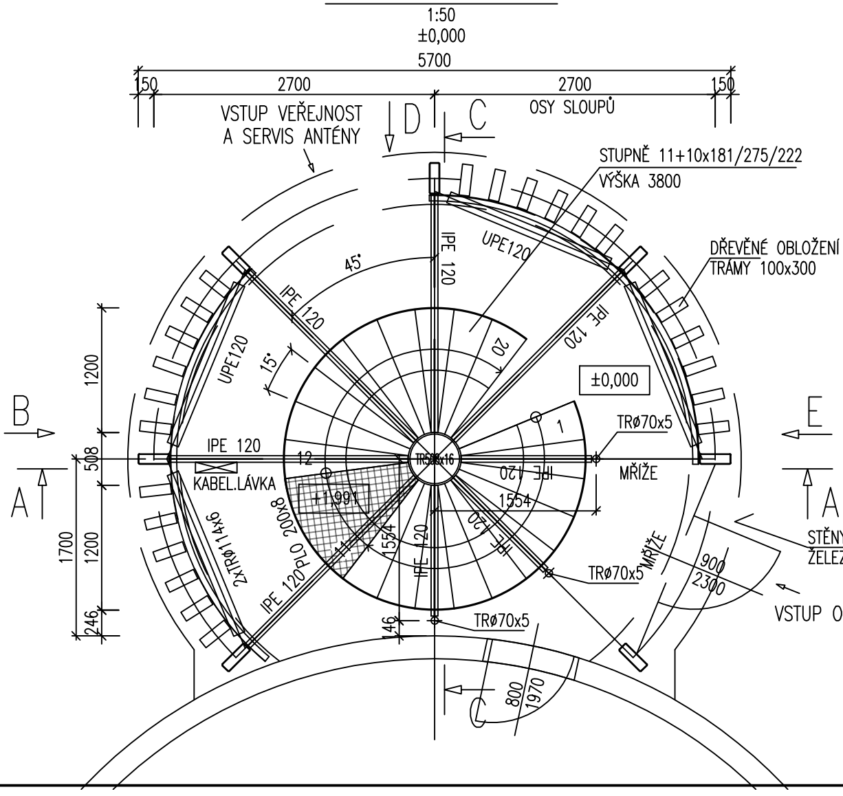
PŮDORYS 1.NP
