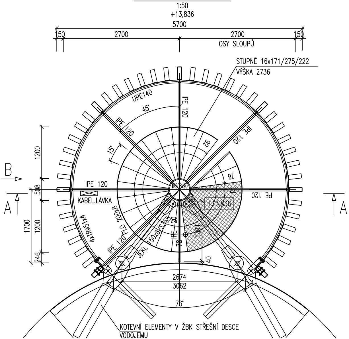
PŮDORYS 4.NP
