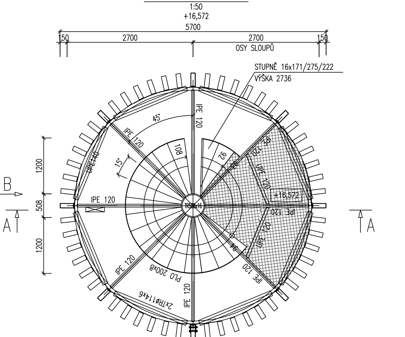
PŮDORYS 6.NP
