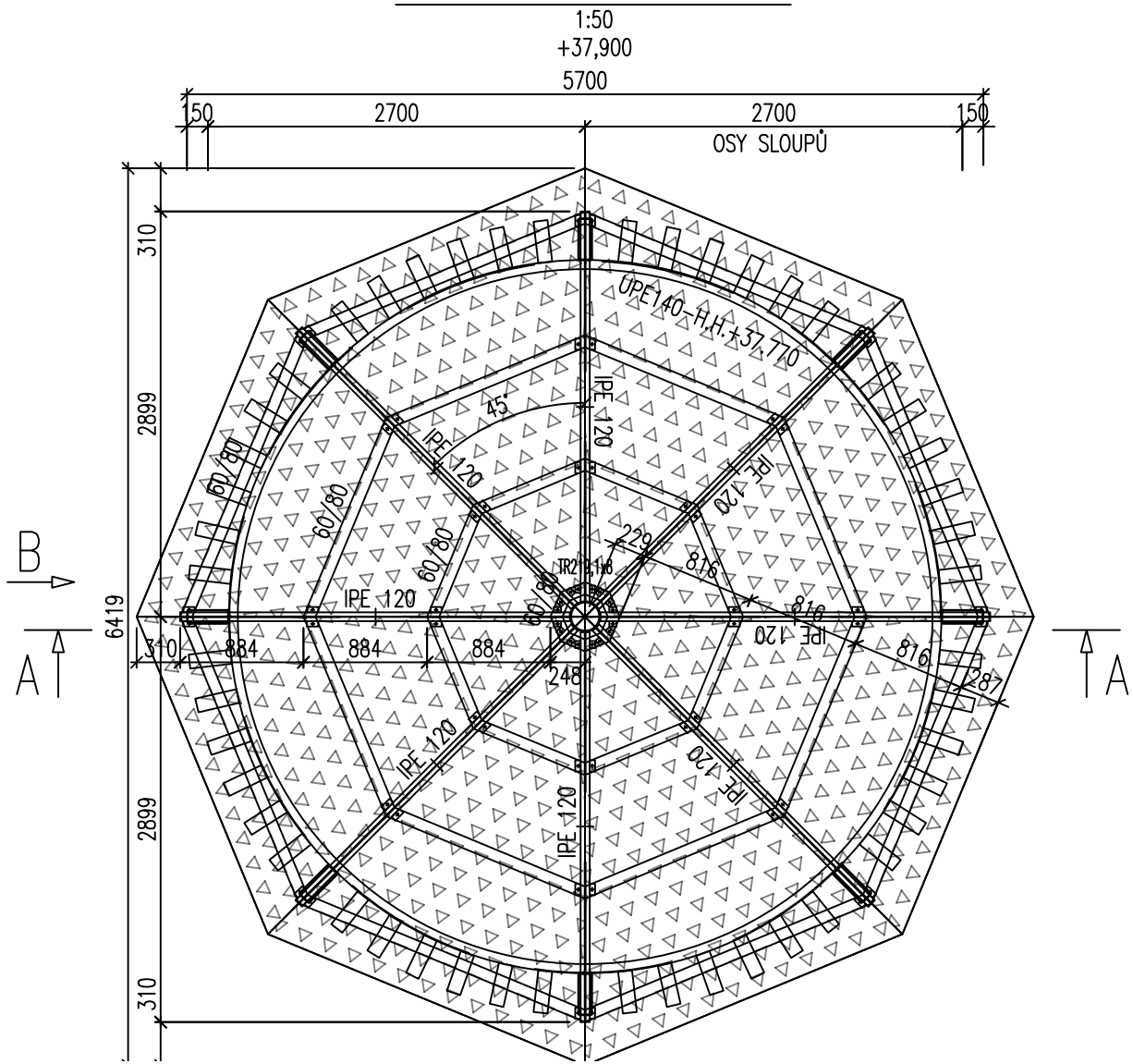
PŮDORYS 13.NP-TECHNOLOGIE
