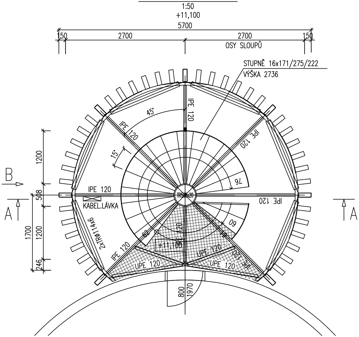
PŮDORYS 3.NP
