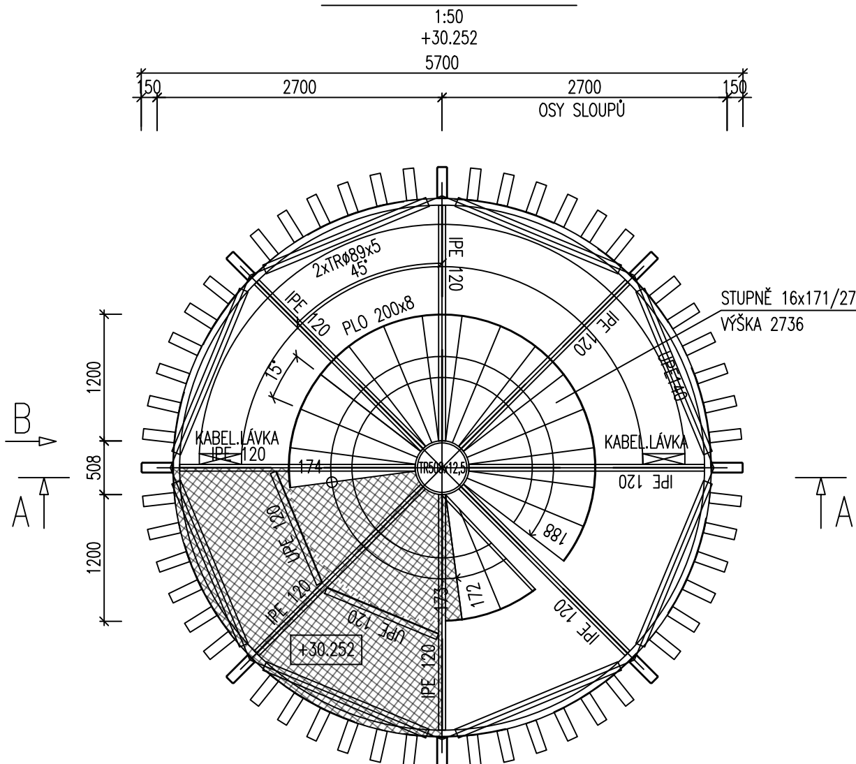
PŮDORYS 11.NP
