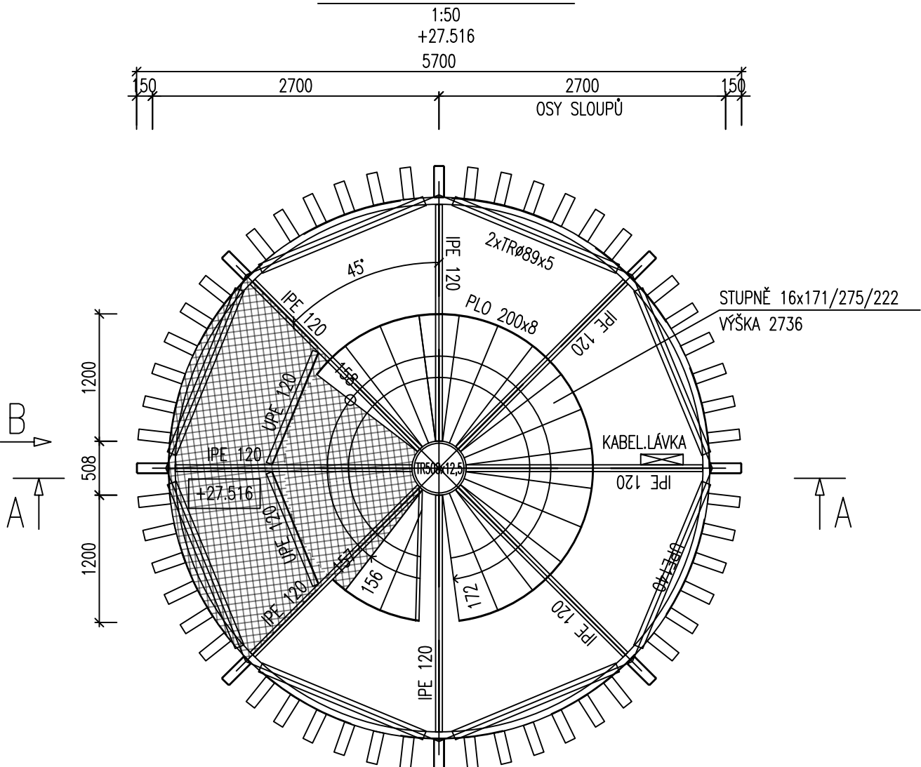
PŮDORYS 10.NP
