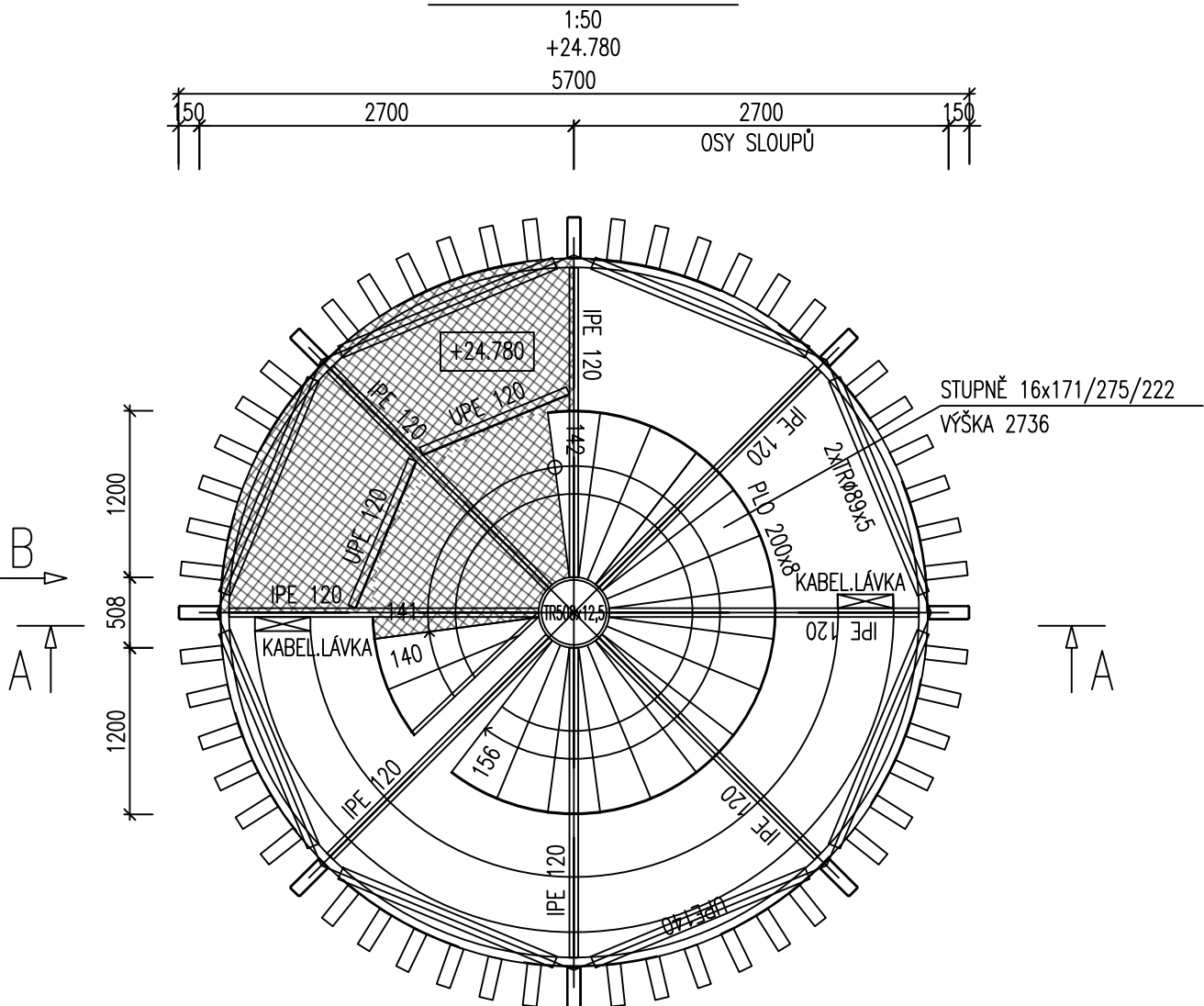
PŮDORYS 9.NP
