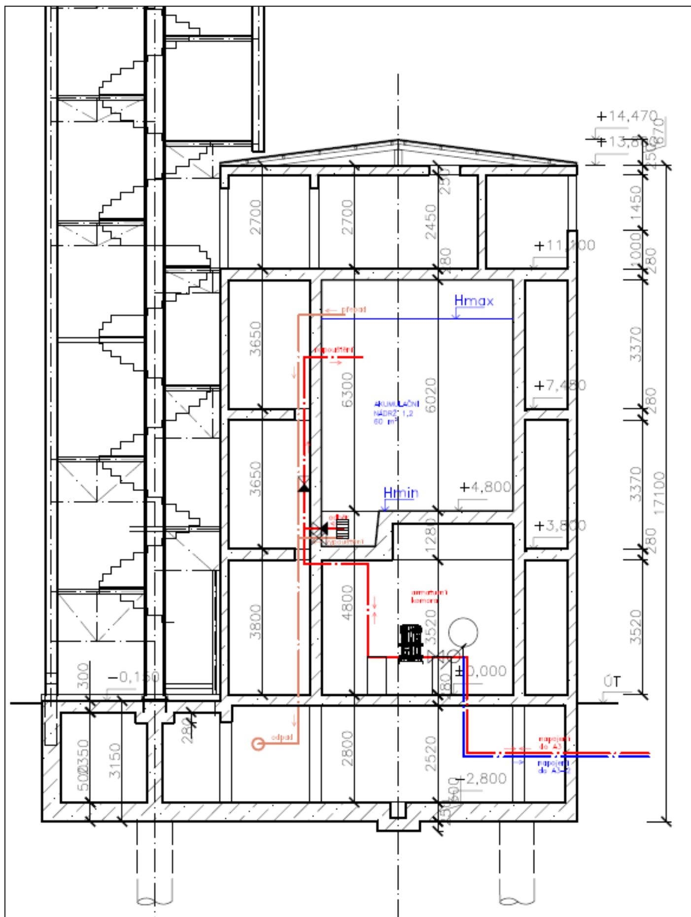
Konstrukční výkres vodojemu včetně základových patek (pilotů) a spodního dílu anténní věže.
